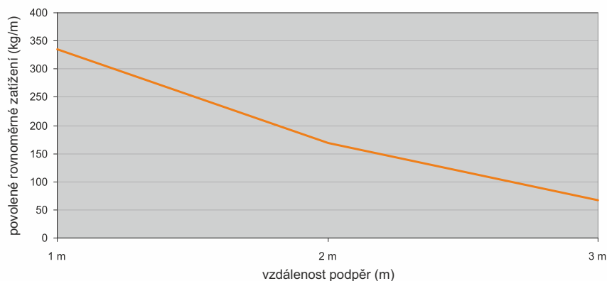
Graf znázorňuje maximální povolené rovnoměrné zatížení žlabu v závislosti na vzdálenosti podpěr
